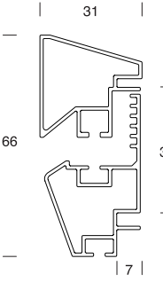
作品厚: 38mm まで UVアクリル: 2mm 見え幅: 31mm 立ち上がり: 66mm フラットパーツ付き (P10 ページ参照)
