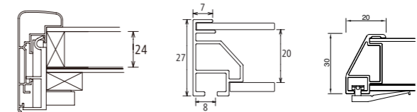
ボルドー断面図
