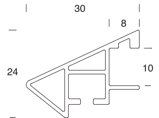
作品厚：5mmまで UVアクリル：2mm 見え幅：30mm カカリ：8mm 立ち上がり：24mm 深さ10mm
