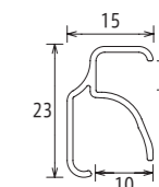
断面図
