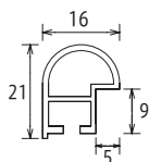
断面図
