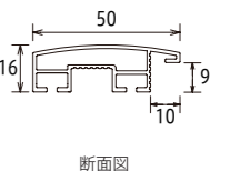
断面図
