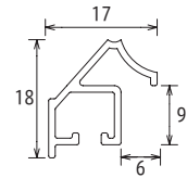
断面図
