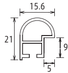
断面図
