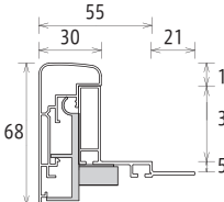
断面図
